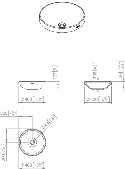
lavabo semi-incasso · Integriertes Becken · Полувстроенная умывальная раковина Ø40 · 12,7h
